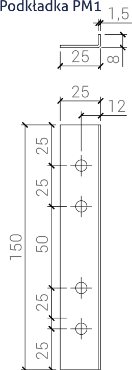
Podkładka PM1
