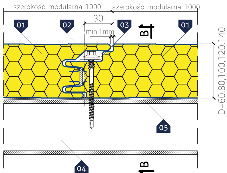
Przekrój B-B
