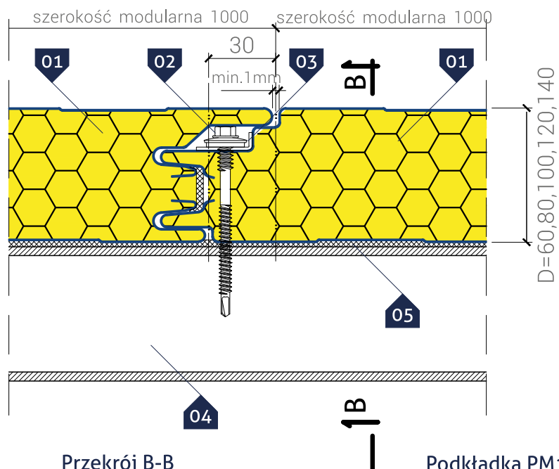
Przekrój A-A
