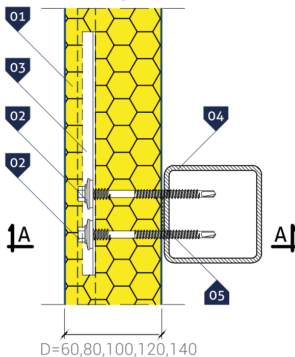
Przekrój B-B
