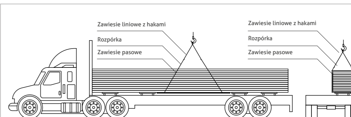
Rys.6 Rozładunek za pomocą zawiesia dla płyt z rdzeniem wełnianym do długości 6,5 m oraz dla płyt z rdzeniem PIR do długości 7,5 m.
