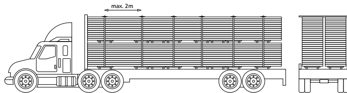
Rys.1 Sposób mocowania pakietów płyt warstwowych na środku transportu.
