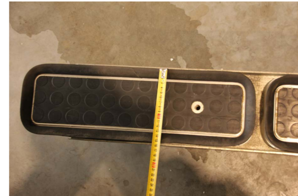
Zdjęcie nr 5. Dopuszczalna maksymalna szerokość przyssawki 15 cm.
