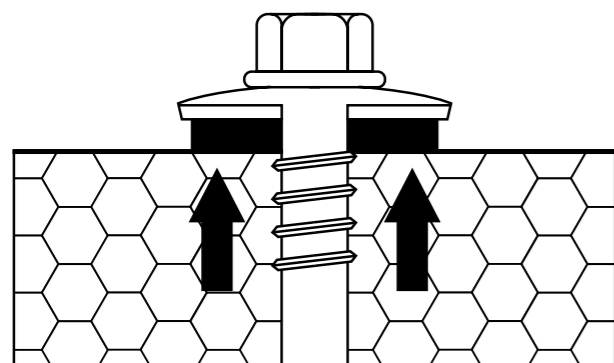
Rys. 10. Prawidłowe zamocowanie łącznika.
