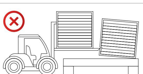
Rys.4 Zwrócić uwagę na długość widel wózka. Zbyt długie widły mogą spowodować uszkodzenie sąsiedniego pakietu płyt warstwowych.
