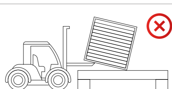
Rys.3 Zwrócić uwagę na długość widel wózka. Zbyt krótkie widły mogą spowodować upadek pakietu płyt warstwowych.
