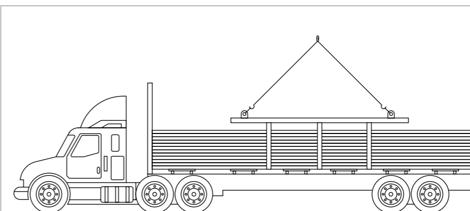
Rys.7 Rozładunek za pomocą zawiesia płyt warstwowych z rdzeniem wełnianym powyżej długości 6,5 m oraz dla płyt z rdzeniem PIR powyżej długości 7,5 m.
