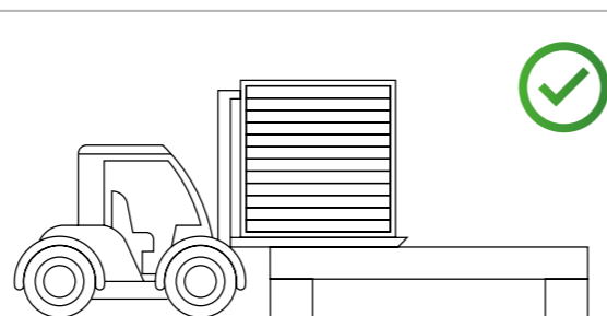
Rys.2 Wózek do rozładunku pakietów płyt warstwowych musi być wyposażony w widły z pionowymi nakładkami zabezpieczającymi krawędzie płyt przed uszkodzeniami.
