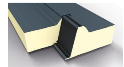
Zamek dla płyty dachowej GS PIR D
